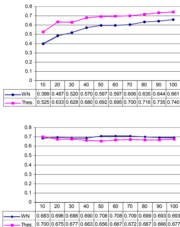
Figura 16. Precisión y cobertura usando distintos porcentajes de cuentas de tripletas (0–100%)
